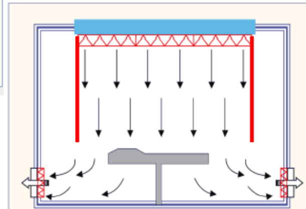
Flux laminaire salle d'opération
