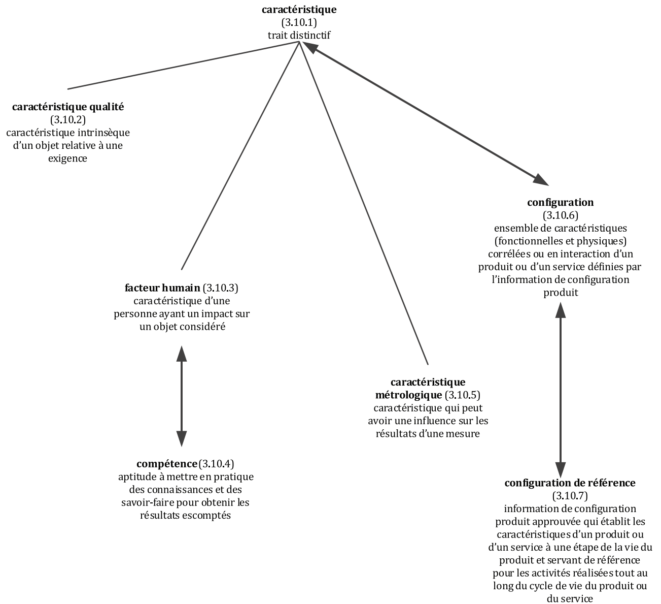
Figure A.13 — 3.10 Concepts de la classe «caractéristiques» et concepts associés
