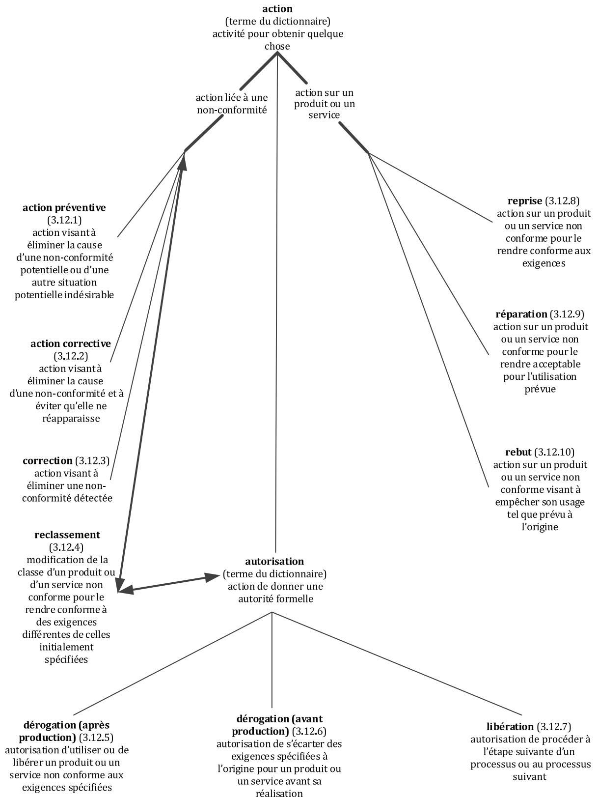
Figure A.15 — 3.12 Concepts de la classe «action» et concepts associés
